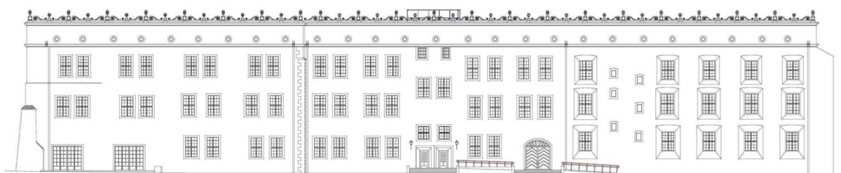
Elewacja północna
