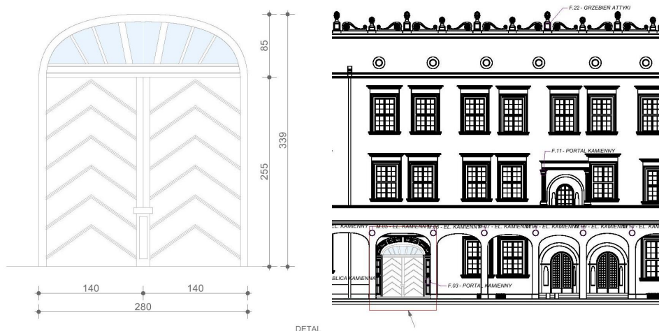
Projekt bramy
